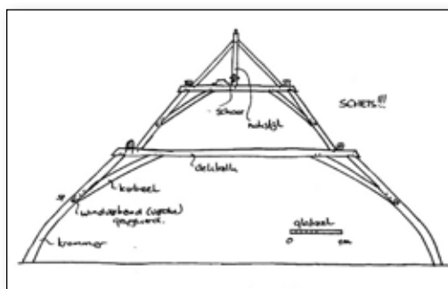
Documentatieschets om een beeld te geven van de verbindingsmiddelen en de typologie. Twee gestapelde dekbalkgebinten. De beide onderste spantbenen zijn ‘krommers’. Op het bovenste dekbalkgebint staat de nokstijl die met andere nokstijlen de nokbalk draagt. (Schets uit Rapport BAAC)
