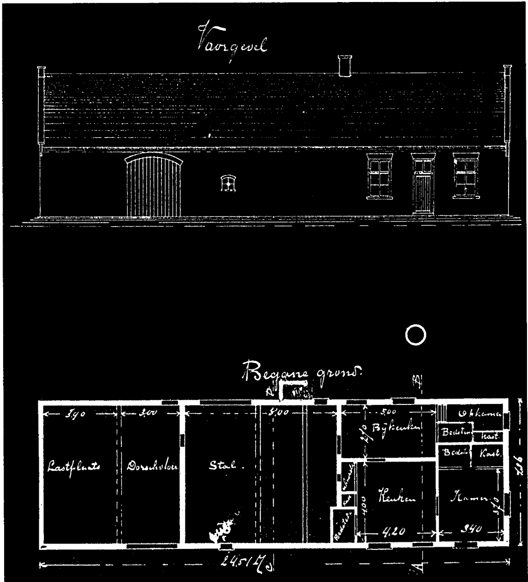
Bouwtekeningen van het boerderijtje aan de Verrehei, waarvoor B & W van Gemert op 3 maart 1908 de bouwvergunning verleende.
