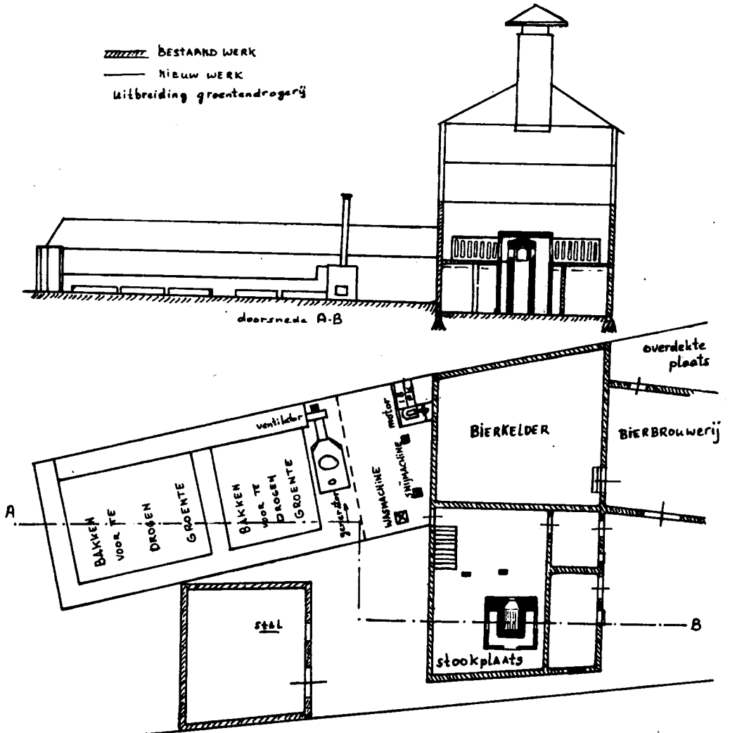
Een gedeelte van de tekeningen die gevoegd waren bij de hinderwetaanvraag voor de oprichting van de groentendrogerij van Swinkels in 1916. (nagetekend van een blauwdruk)
